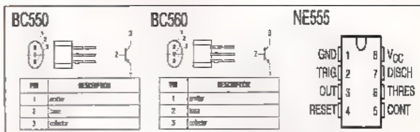
Voor de duidelijkheid \blacksquare van de transistoren en de 555 de pinbezetting gegeven
